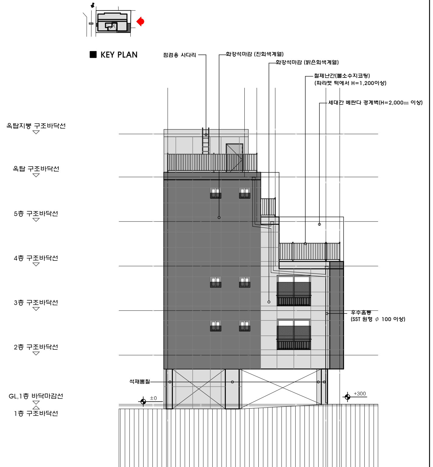
동측면도 축척:1/150
