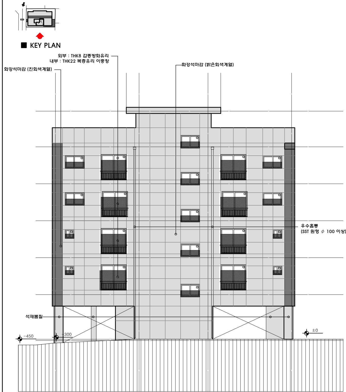
남측면도 축척:1/150
