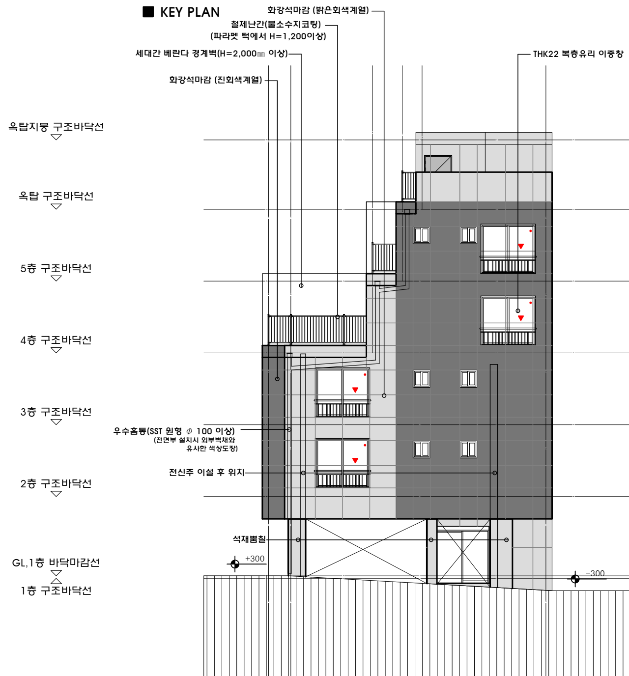
서측면도 축척:1/150
