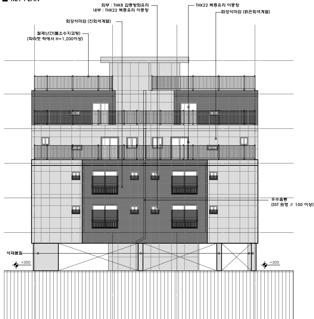
북측면도 축척:1/150
